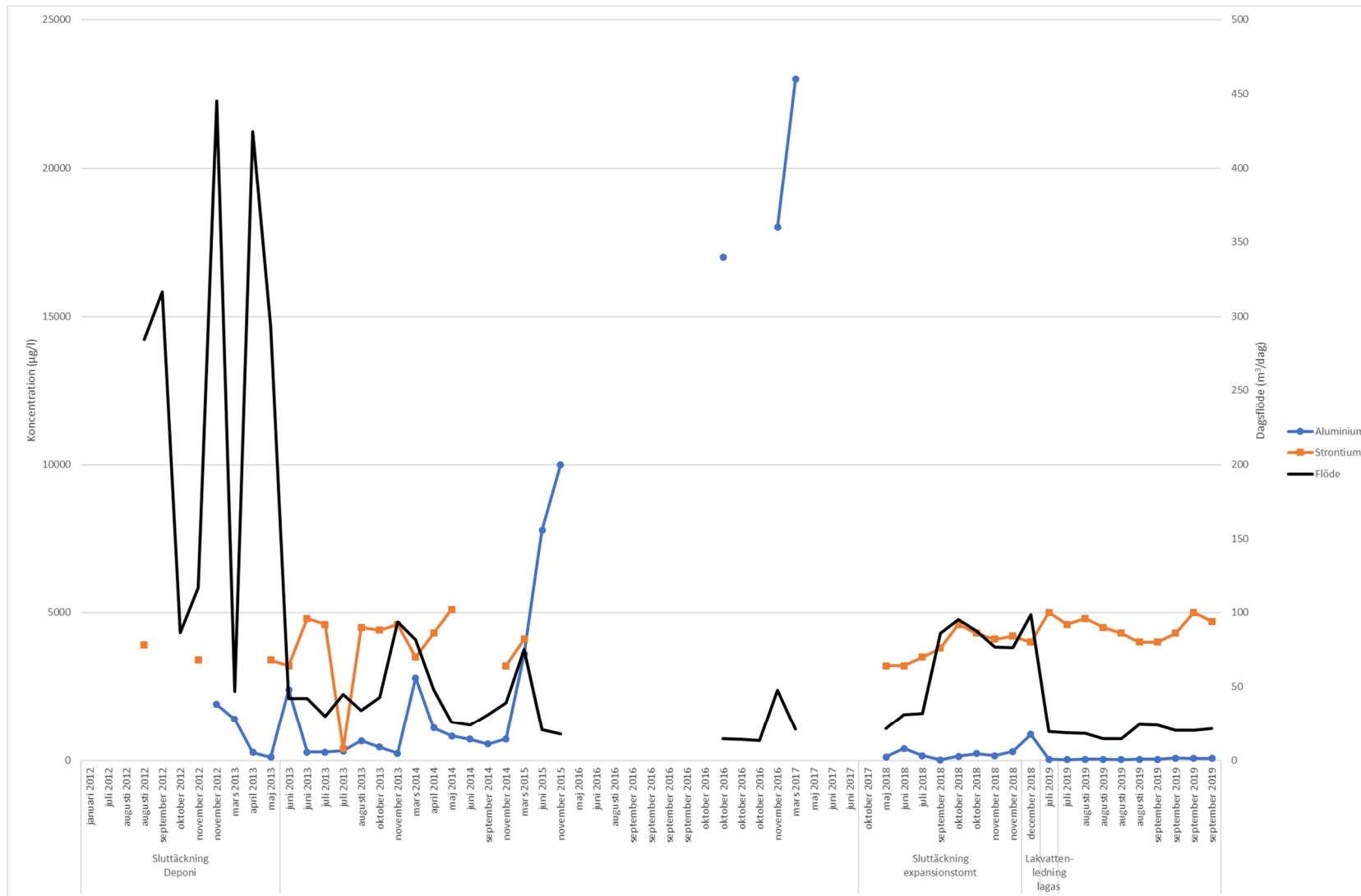
Figur 3 Aluminium och strontium (µg/l). Flöden i m³/dygn.
