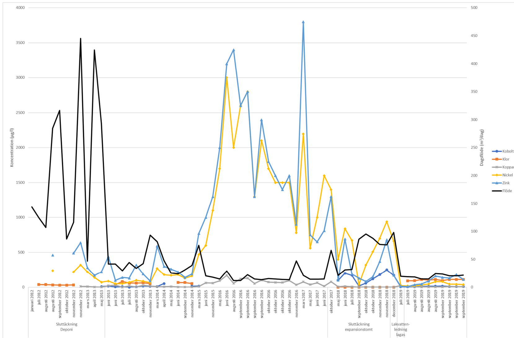
Figur 2. Kobolt (Co), Koppars (Cu), Nickel (Ni), Zink (Zn) (ug/l). Flöden i m 3 /dygn.
